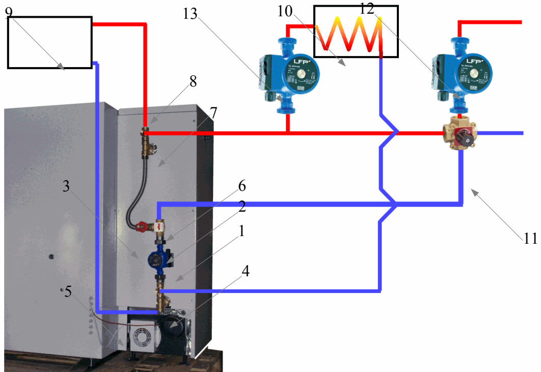
Rys nr 19. Opis schematyczny Grupy hydraulicznej z zaworem termostaticznym TV pracującej w otwartym układzie grzewczym:
