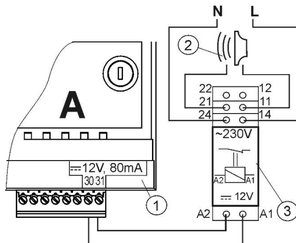
Rys. 35 Podłączenie zewnętrznego urządzenia alarmowego, gdzie: 1- regulator moduł A, 2 - zewnętrzne urządzenie alarmowe, 3 - moduł U3.
