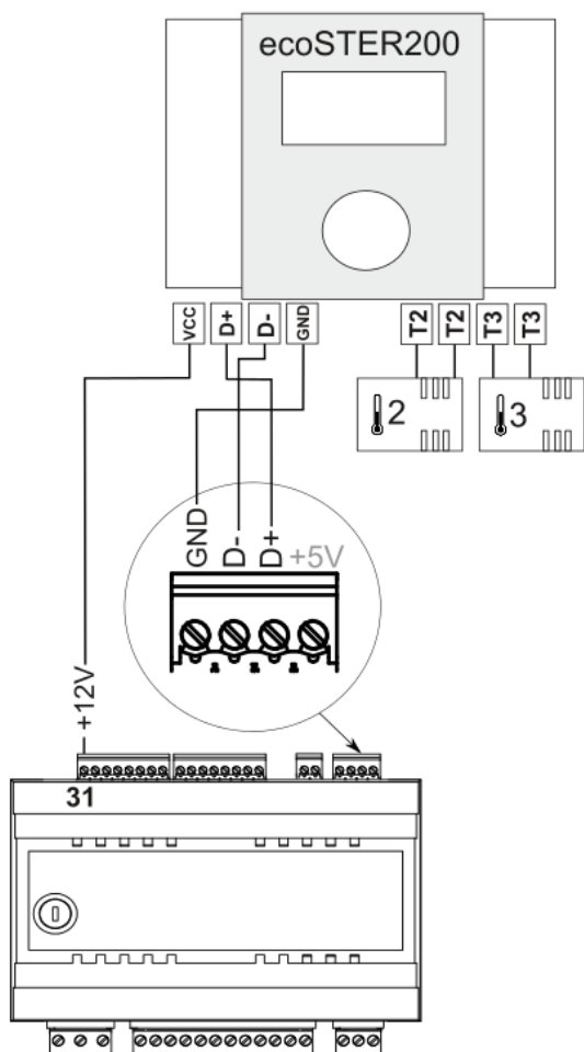
Rys. 36 Schemat podłączenia elektrycznego (czteroprzewodowego) ecoSTER200 z modulem A regulatora.
