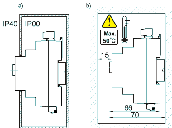
Rys. 25 Metody zabudowy modułów: a – w obudowie modułowej z dostępem do powierzchni czołowej, b – w obudowie bez dostępu do powierzchni czołowej.
