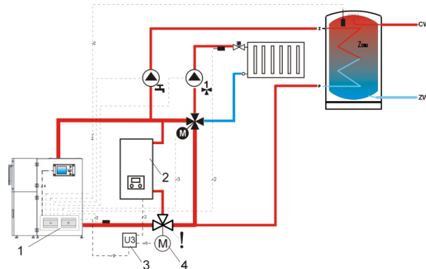
Rys. 33 Schemat hydrauliczny z kotłem rezerwowym i zaworem czterodrogowym w obiegu zamkniętym, gdzie: 1 – regulator ecoMAX, 2 – kocioł rezerwowy, 3 – moduł U3, 4 – siłownik zaworu przełączającego (z wyłącznikami krańcowymi). Uwaga: aby zapewnić swobodny przepływ grawitacyjny wody w obiegu kotła, przekrój czynnika zaworu przełączającego (4) musi być większy, bądź równy przekrojowi rury obiegu kotła. Stosować duże przekroje rur grawitacyjnego obiegu kotła.
