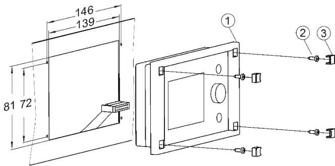
Rys. 20 Zainstalowanie panelu w płycie montażowej, gdzie: 1- panel sterujący, 2 - blachowkręt 2.9x13, 3 - zaślepka.
