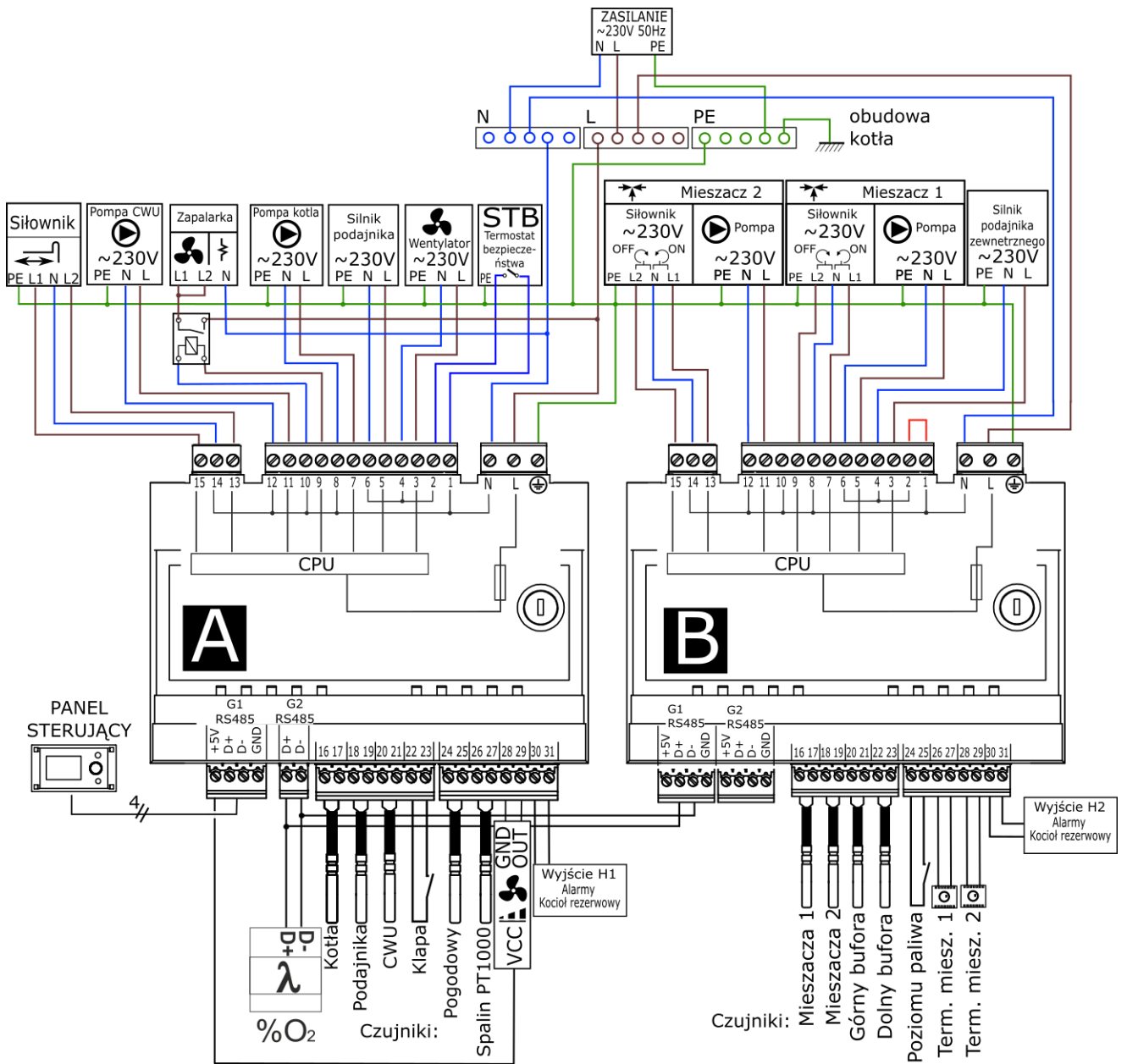
Rys. 27 Schemat połączeń elektrycznych dla modułu A i B.
