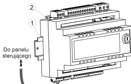
Rys. 23 Osadzenie regulatora na szynie, gdzie: 1 - szyna DIN TS35, 2 - zaczepy.
