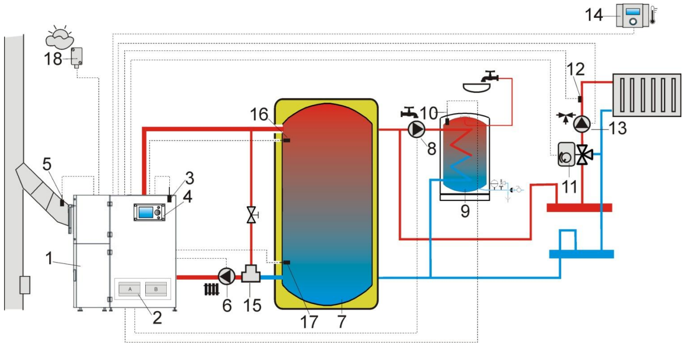
Rys. 17 Schemat z buforem ciepła 2 , gdzie: 1 – kocioł, 2 – regulator, 3 – czujnik temperatury kotła, 4 – panel sterujący regulatora, 5 – czujnik temperatury spalin, 6 – pompa kotła, 7 – bufor ciepła, 8 – pompa obiegu ciepłej wody użytkowej, 9 - zasobnik ciepłej wody użytkowej, 10 – czujnik temperatury ciepłej wody użytkowej, 11 – siłownik elektryczny mieszacza, 12 – czujnik temperatury mieszacza, 13 – pompa obiegu mieszacza, 14 – panel pokojowy z funkcją termostatu pokojowego ecoSTER200, 15 – termostacyjny zawór trójdrogowy, 16 – czujnik temperatury bufora górny, 17 – czujnik temperatury bufora dolny, 18 – czujnik temperatury pogodowy.
