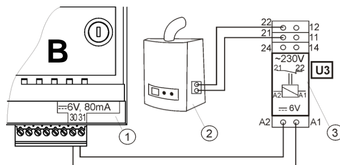
Rys. 30 Przykładowy schemat układu do podłączenia kotła rezerwowego do regulatora, gdzie: 1- regulator moduł B, 2 – kocioł rezerwowo (gazowy lub olejowy), 3 – Moduł U3 składający się z przekaźnika RM 84-2012-35-1006 i podstawki GZT80 RELPOL.
