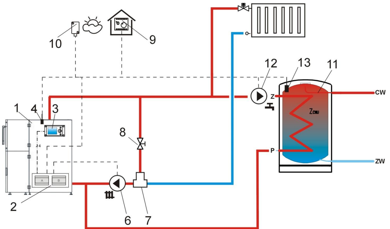
Rys. 18 Schemat z termostatycznym zaworem trójdrogowym chroniącym temperaturę wody powrotnej 3 , gdzie: 1 – kocioł z podajnikiem, 2 – regulator, 3 – panel sterujący regulatora, 4 – czujnik temperatury kotła, 6 – pompa obiegu centralnego ogrzewania, 7 – termostatyczny zwór trójdrogowy, 8 – zawór dławiący (grzybkowy), 9 – termostat pokojowy, 10 – czujnik temperatury pogodowej, 11 – zasobnik ciepłej wody użytkowej, 12 – pompa obiegu ciepłej wody użytkowej, 13 – czujnik temperatury ciepłej wody użytkowej.
