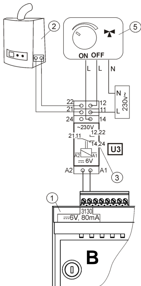
Rys. 34 Schemat elektryczny sterowania zaworem przełączającym kotła rezerwowego, gdzie: 1 – regulator moduł B, 2 – kocioł rezerwowy, 3 – moduł U3, 5 – siłownik zaworu przełączającego (z wyłącznikami krańcowymi), uwaga: zaciski 22,21,24 muszą być odseparowane galwanicznie od zacisków 12,11,14.
