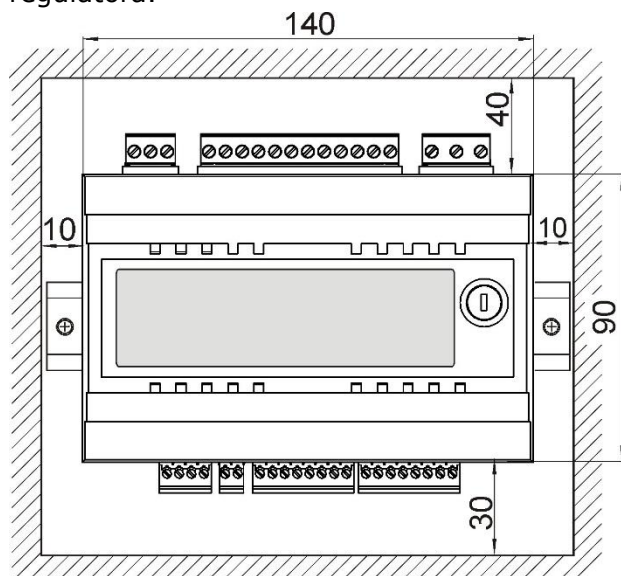
Rys. 24 Warunki zabudowy pojedynczego modułu.
