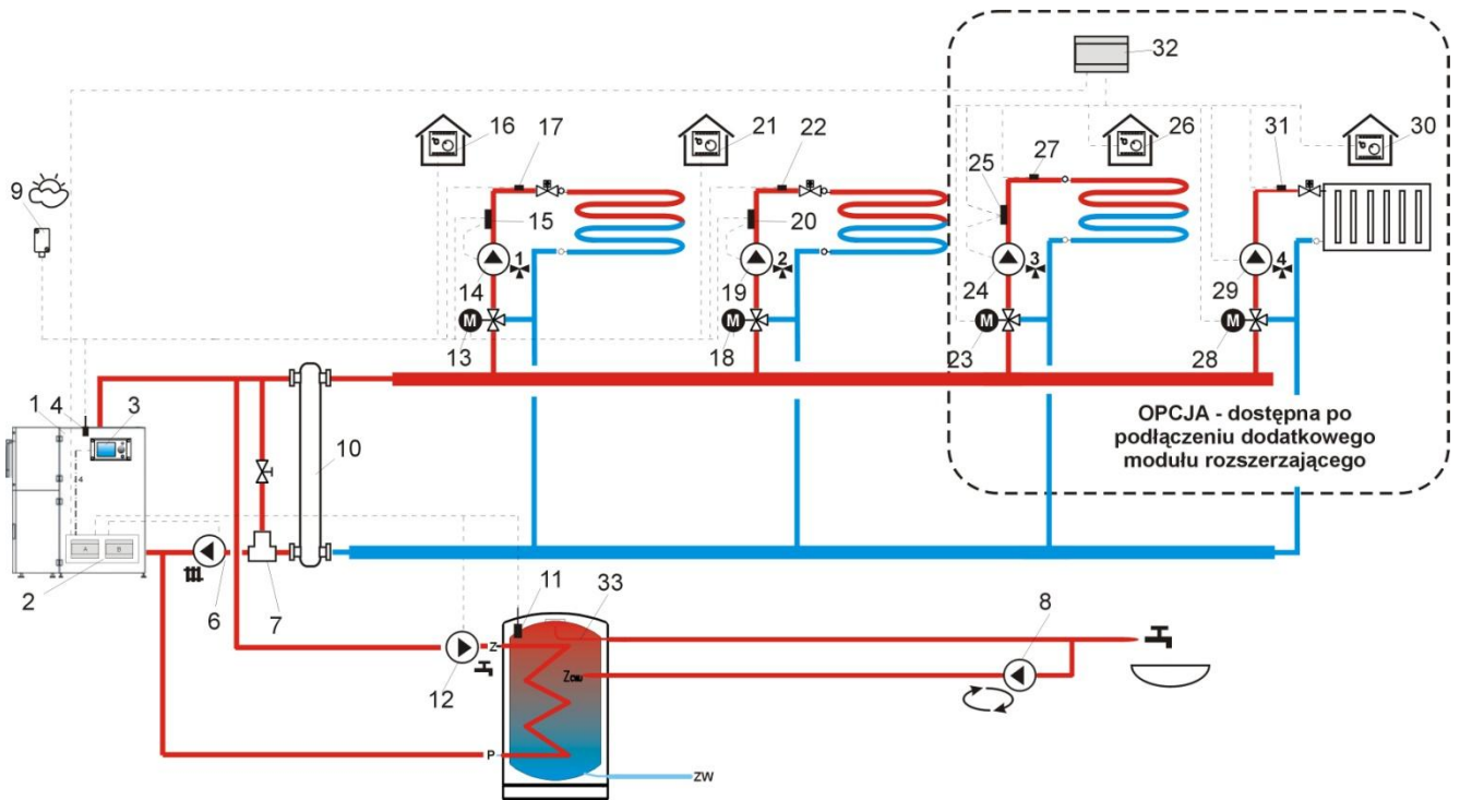
Rys. 19 Schemat z termostatycznym zaworem trójdrogowym chroniącym temperaturę wody powrotnej i dwoma zaworami trójdrogowymi zasilającymi ogrzewanie podłogowe oraz z dwoma dodatkowymi obiegami mieszacza po podłączeniu modułu dodatkowego 4 , gdzie: 1 – kocioł, 2 – regulator, 3 – panel sterujący regulatora, 4 – czujnik temperatury kotła, 6- pompa obiegu centralnego ogrzewania, 7 – termostatyczny zawór trójdrożny (w celu ochrony powrotu kotła), 8 – pompa cyrkulacyjna, 9 -czujnik temperatury pogodowy, 10 – sprzęgło hydrauliczne (zapewnia brak konieczności równoważenia przepływów pomp), 11 – czujnik temperatury CWU, 12 – pompa obiegu ciepłej wody użytkowej, 13 – siłownik mieszacza 1, 14 – pompa obiegu mieszacza 1, 15 – zewnętrzny termostat zabezpieczający ogrzewanie podłogowe 55 °C (odcina zasilanie elektryczne pompy mieszacza po przekroczeniu maksymalnej temperatury – termostat nie wchodzi w skład wyposażenia regulatora), 16 – termostat pokojowy mieszacza 1, 17 – czujnik temperatury mieszacza 1, 18 – siłownik mieszacza 2, 19 – pompa obiegu mieszacza 2, 20 – zewnętrzny termostat zabezpieczający ogrzewanie podłogowe 55 °C, 21 – termostat pokojowy mieszacza 2, 22 – czujnik temperatury mieszacza 2, 23 – siłownik mieszacza 3, 24 – pompa obiegu mieszacza 3, 25 – zewnętrzny termostat zabezpieczający ogrzewanie podłogowe 55 °C, 26 – termostat pokojowy mieszacza 3, 27 – czujnik temperatury mieszacza 3, 28 – siłownik mieszacza 4, 29 – pompa obiegu mieszacza 4, 30 – termostat pokojowy mieszacza 4, 31 – czujnik temperatury mieszacza 4, 32 – rozszerzający moduł mieszaczowy, 33 – zasobnik ciepłej wody użytkowej.
