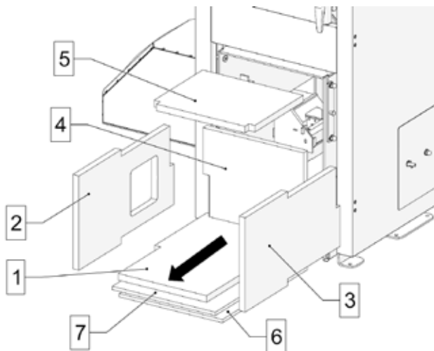
Rys.: Komora ceramiczna EEI Pellets 16kW, 24kW, 32kW
