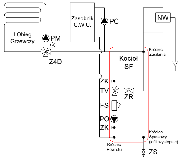
Rys nr 25. Układ otwarty + wymiennik ciepła + CWU po stronie wtórnej + 1 obieg na zaworze 3D
