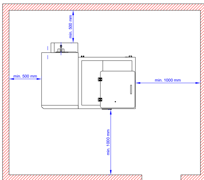
Rys nr 20. Przykład umiejscowienia kotła typu Smart Fire SF41 z zasobnikiem 400L w kotłowni
