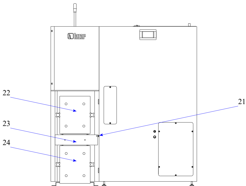
Rys nr 5. Opis schematyczny kotłów typu Smart Fire SF 11, SF15, SF22, SF31 oraz SF41
