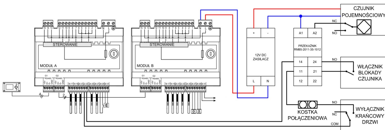
Rys nr 17. Schemat podłączenia pojemnościowego czujnika zblizeniowego
