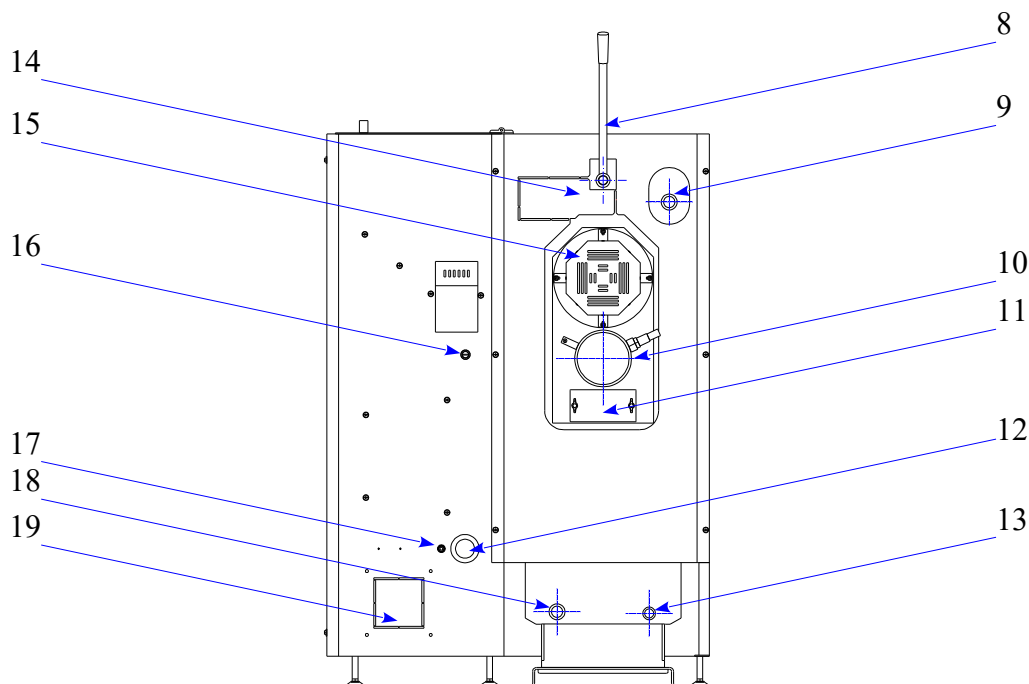
Rys nr 15. Opis schematyczny kotłów typu Smart Fire SF 11, SF15, SF22, SF31 oraz SF41
